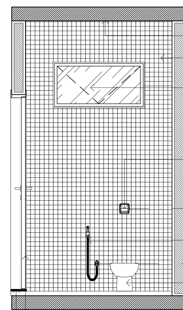
02 VISTA 01 ESC: 1/25
