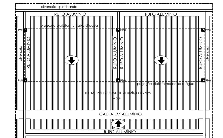
03 PLANTA DE COBERTURA SOB CAIXAS D'ÁGUA ESC: 1/100
